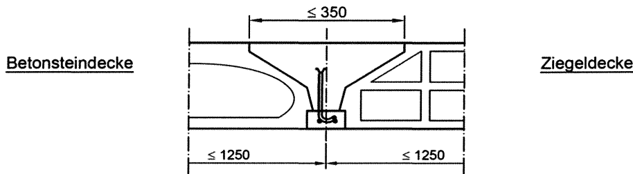
Bild 4: Balkendecke nach Anlage 8, Abschnitt 4
