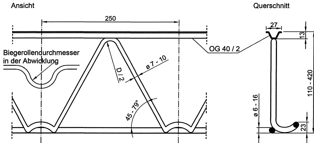
Bild 1: FILIGRAN - SE-Träger
