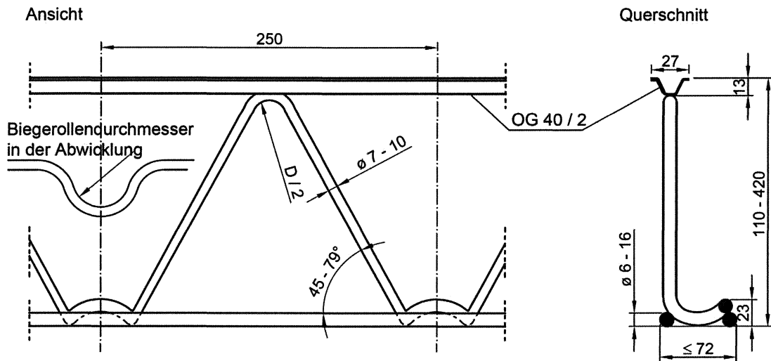
Bild 2: FILIGRAN - S-Träger
