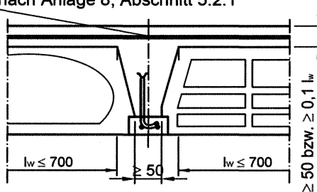
Bild 7: Rippendecke nach Anlage 8, Abschnitt 5
