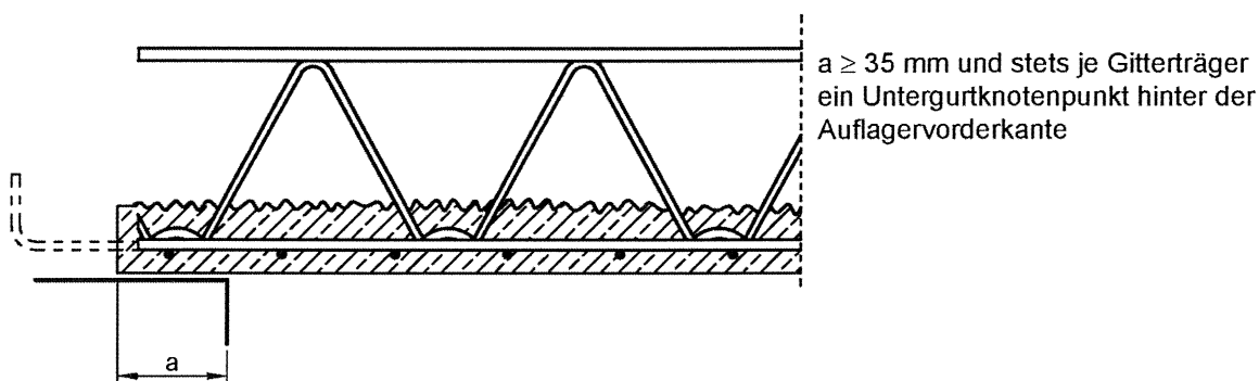
Bild 15: Auflagerung mit Montageunterstützung am Rand
