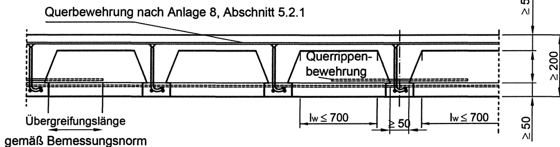
Bild 8: Rippenenelementdecke nach Anlage 8, Abschnitt 5
