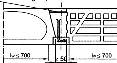
Bild 5: Rippendecke nach Anlage 8, Abschnitt 5
