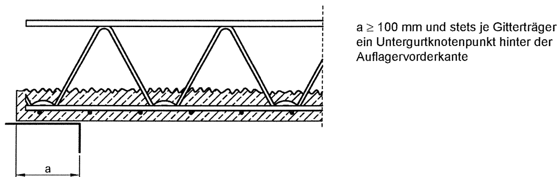
Bild 13: Auflagerung ohne Montageunterstützung am Rand
