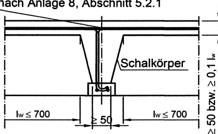
Bild 7: Rippendecke nach Anlage 8, Abschnitt 5
