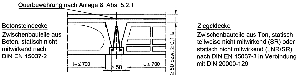
Bild 8: Rippendecke nach Anlage 8, Abschnitt 5
