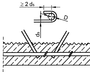
Bild 14: Querbügel
