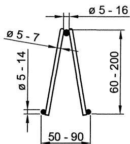
Bild 1: D-Gitterträger
