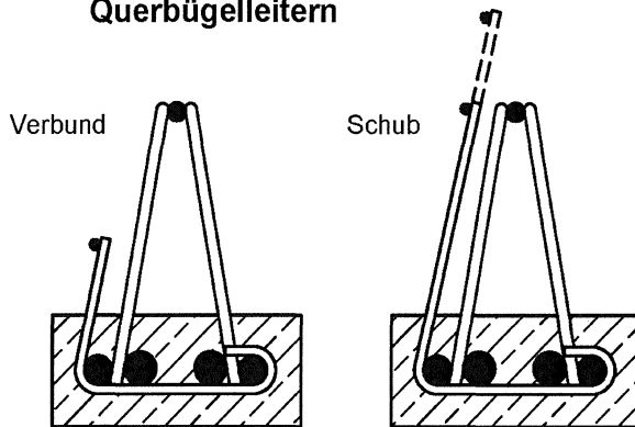
Bild 15: D- / E-Träger mit Betonfußleiste und Querbügelleitern
