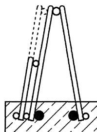
Bild 23: DH- bzw. EH-Gitterträger als Verbund- und Schubzulagen
