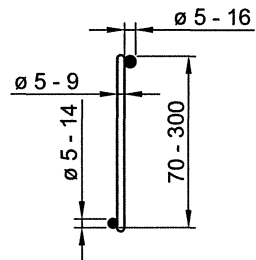
Bild 4: EH-Gitterträger
