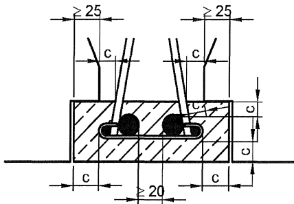
Bild 15: D- / E-Träger mit Betonfußleiste und Querbügelleitern
