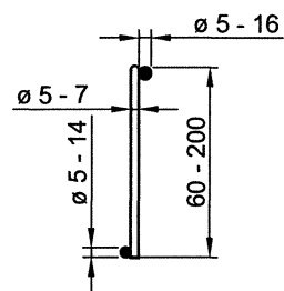
Bild 3: DH-Gitterträger
