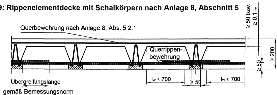
Bild 10: Rippen-elementdecke mit Betonschalung nach Anlage 8, Abschnitt 5
