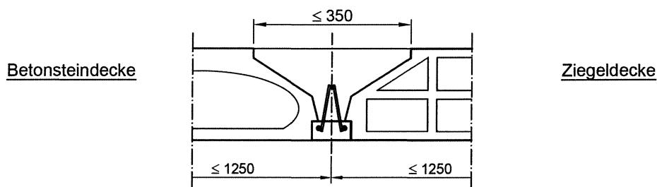
Bild 6: Rippendecke nach Anlage 8, Abschnitt 5
