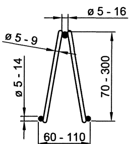
Bild 2: E-Gitterträger
